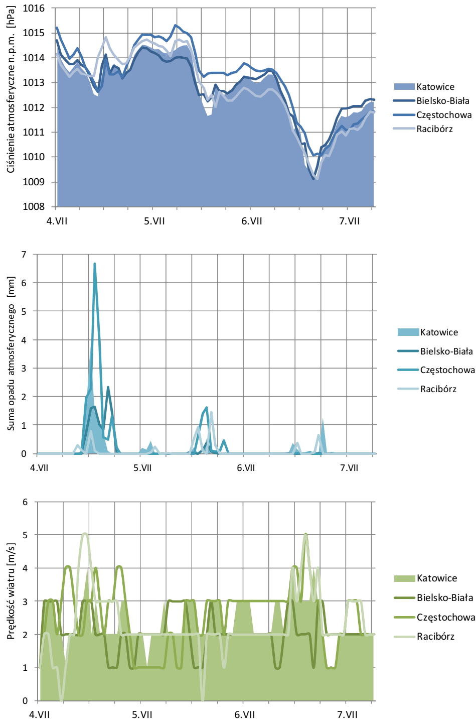
Rys. 2 przedstawia prognozowany przebieg temperatury powietrza, ciśnienia atmosferycznego, prędkości wiatru i opadu atmosferycznego dla Bielska-Białej, Częstochowy, Katowic i Raciborza z modelu COSMO - prognoza od 0 UTC na 78 godzin w przód z krokiem 1-godzinnym (źródło danych: IMGW-PIB Dział Numerycznych Prognoz Meteorologicznych COSMO).
